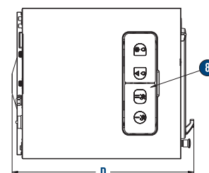
TOP ELEVATION
